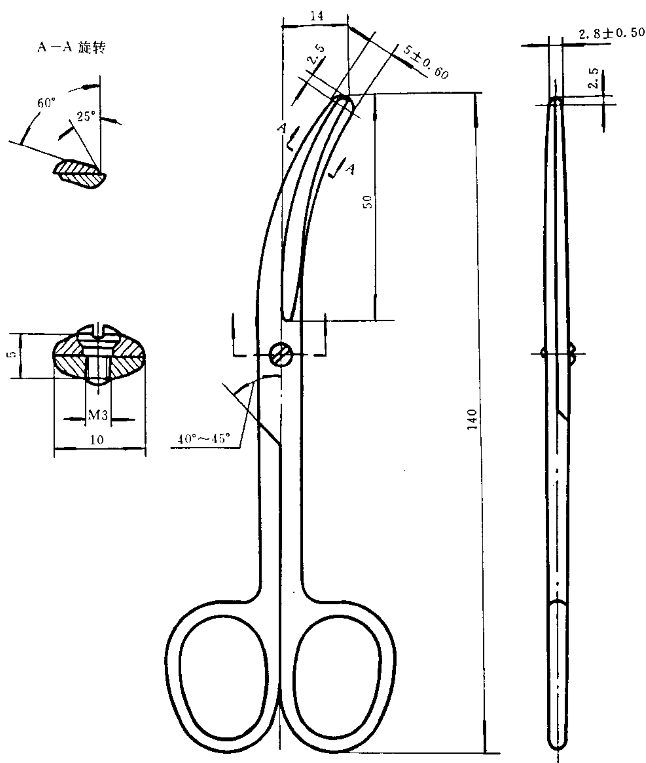
图1 脐带剪
