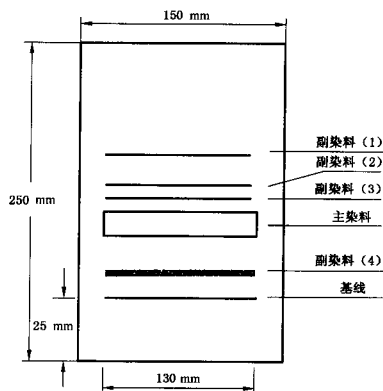
图 1 副染料纸上层析示意图
