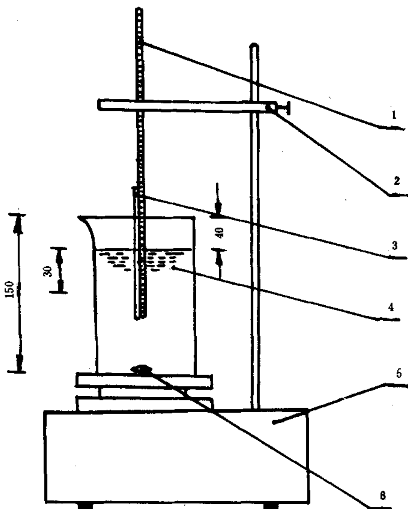
图 1 熔点测定装置
